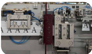
CUTTING DIE
